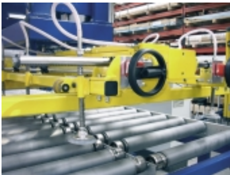
Breitenverstellung mit Handrad oder Motor
