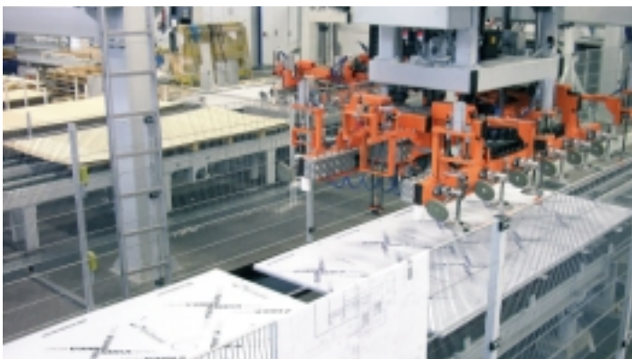
vollautomatisches 2-Achs-Portal
