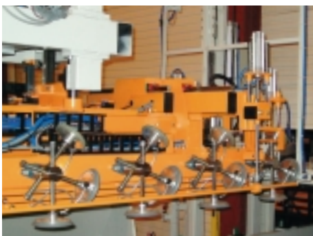
vollautomatischer Saugerwechsel
